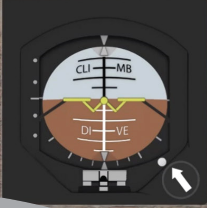
Attitude Indicator (ADI)
